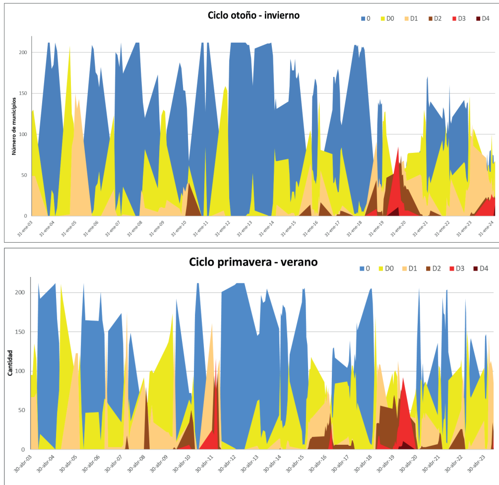
Figura 2. Niveles de sequía registrados en los municipios de Veracruz desde el 2003 hasta abril del 2024.
