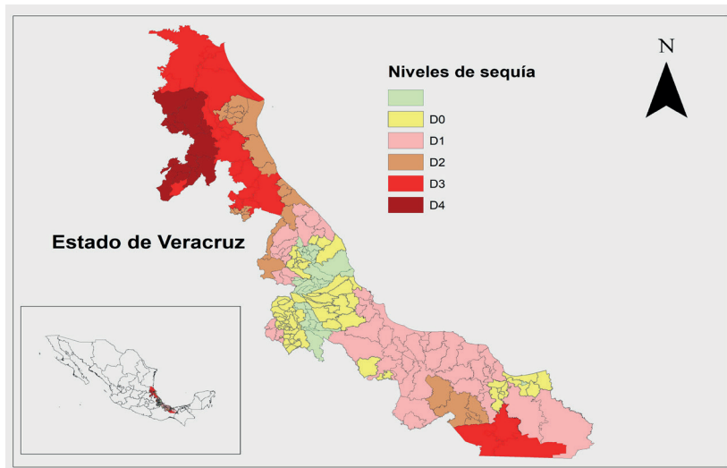
Figura 3. Niveles de sequía registrados por el Monitor de Sequía de México a marzo del 2024 para los municipios del estado de Veracruz.
